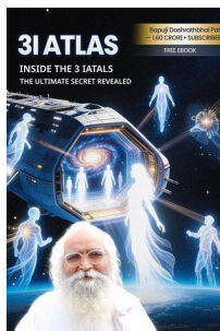
3i Atlas
